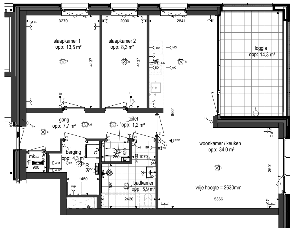
Plattegrond 1 : 100
