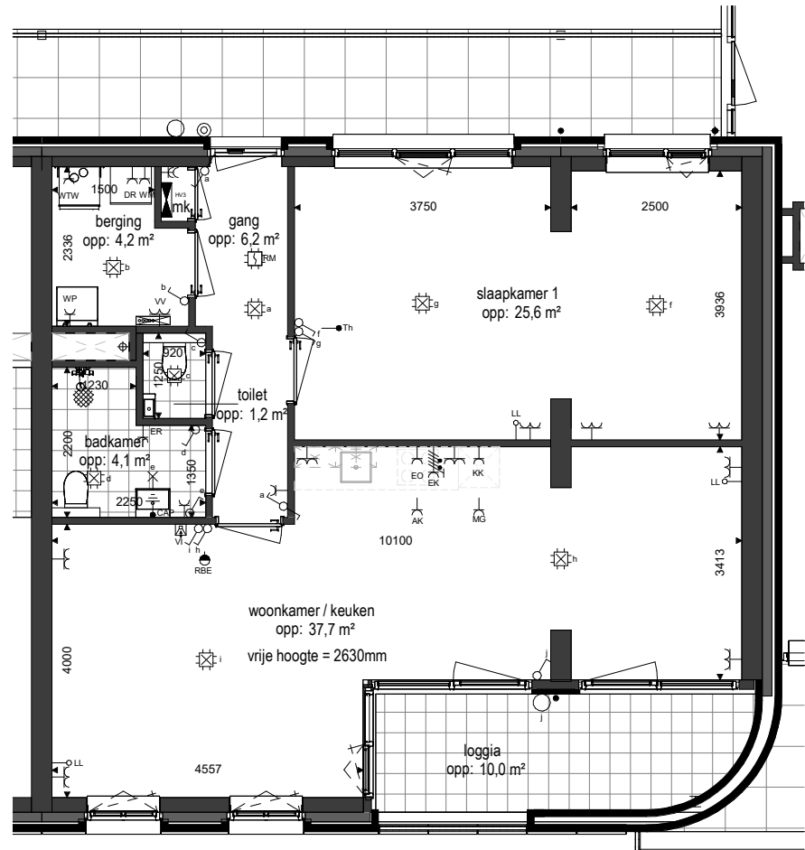
Plattegrond 1 : 100
