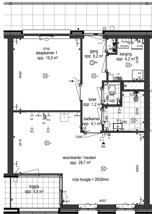
Plattegrond 1 : 100
