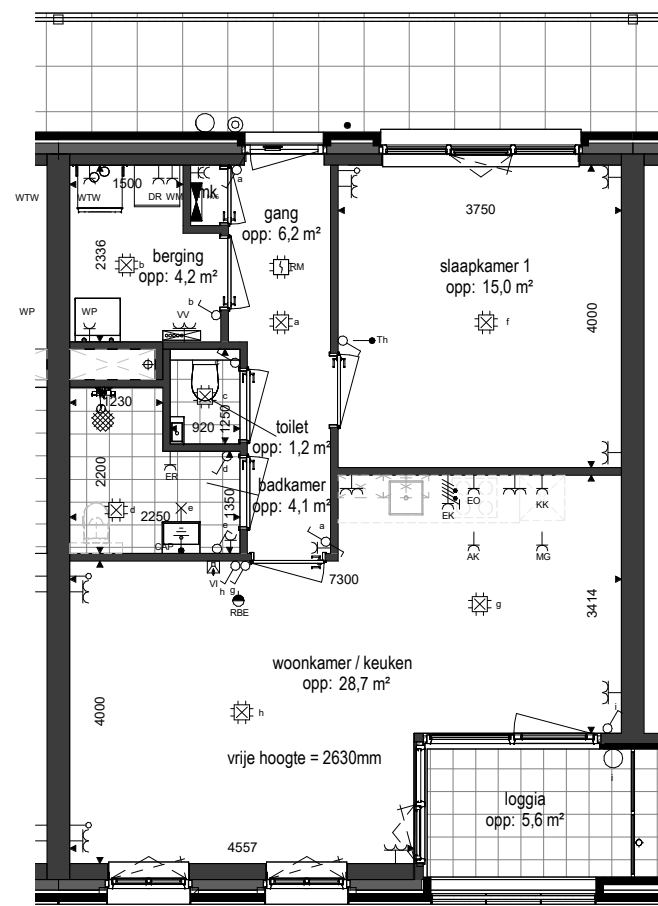
Plattegrond
