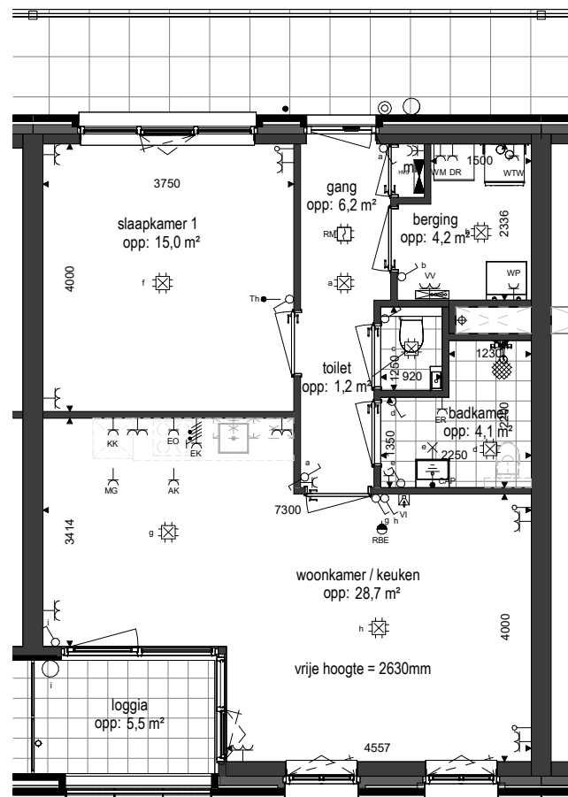
Begane grond 1 : 100
