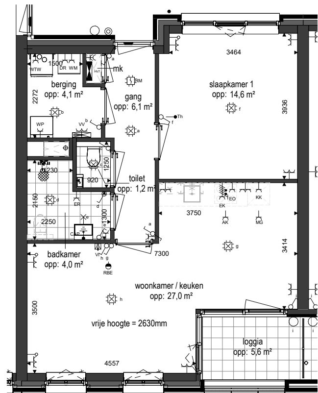
Plattegrond 1 : 100
