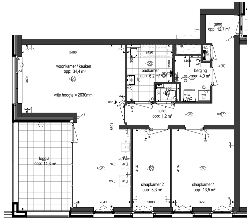
Begane grond 1 : 100
