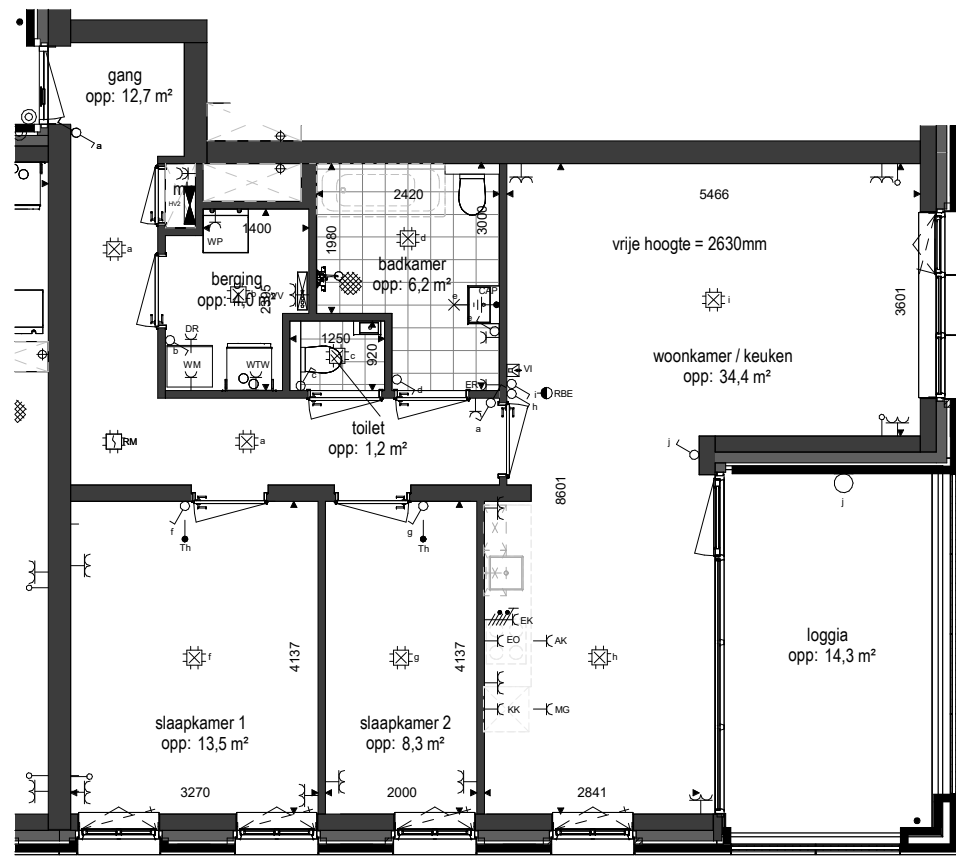
Plattegrond 1 : 100
