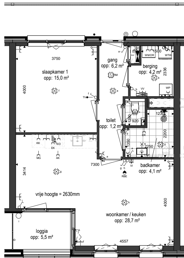
Plattegrond 1 : 100
