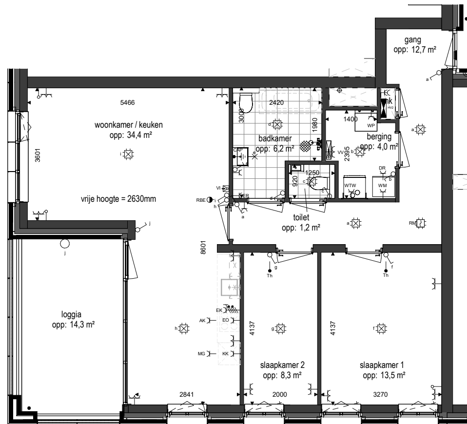
Plattegrond 1 : 100
