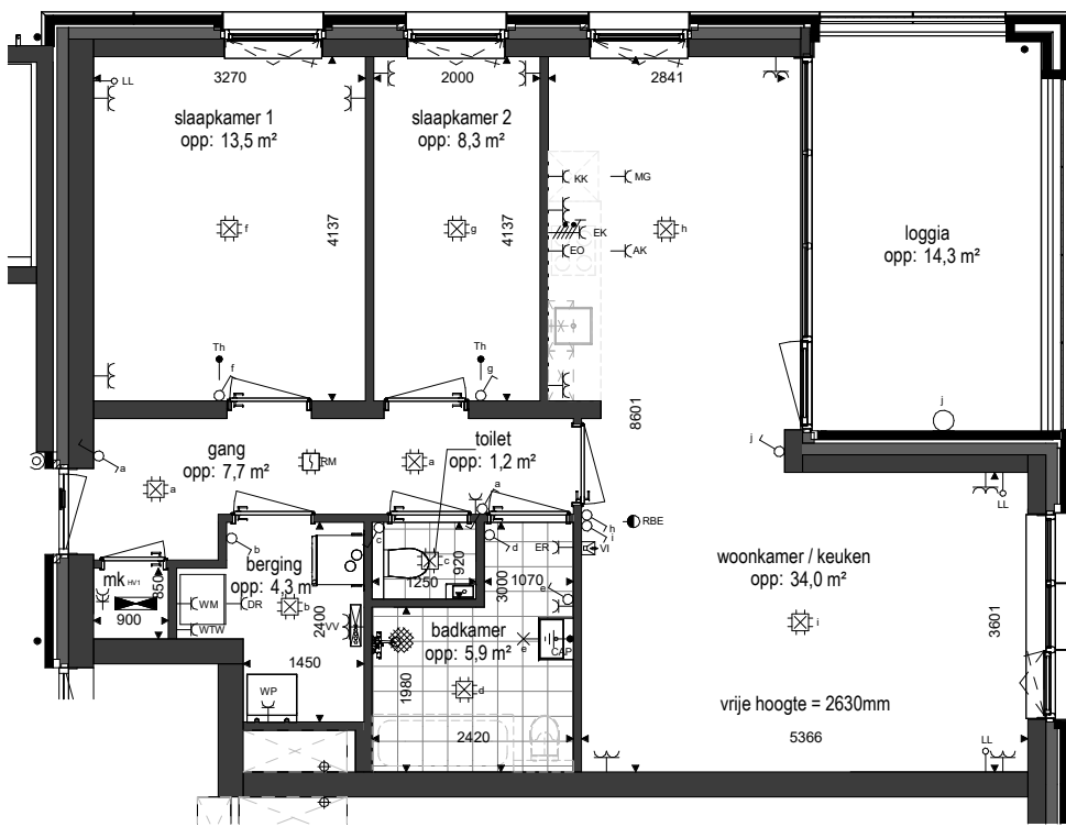
Tweede verdieping 1 : 100
