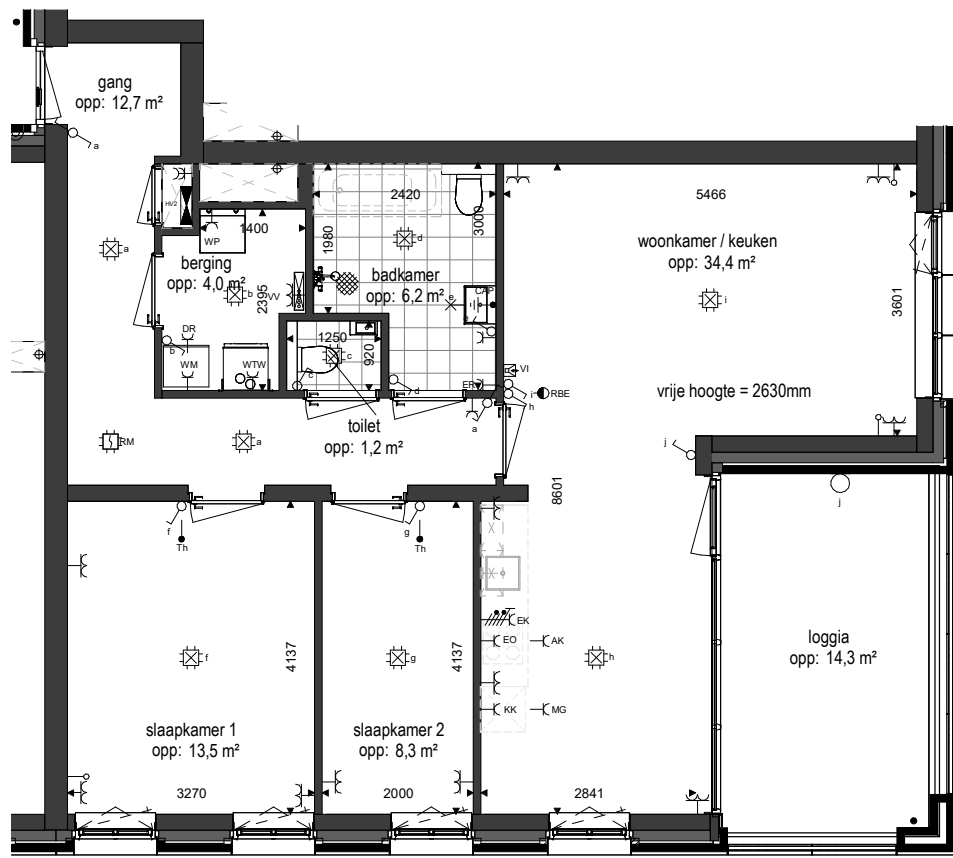
Plattegrond
