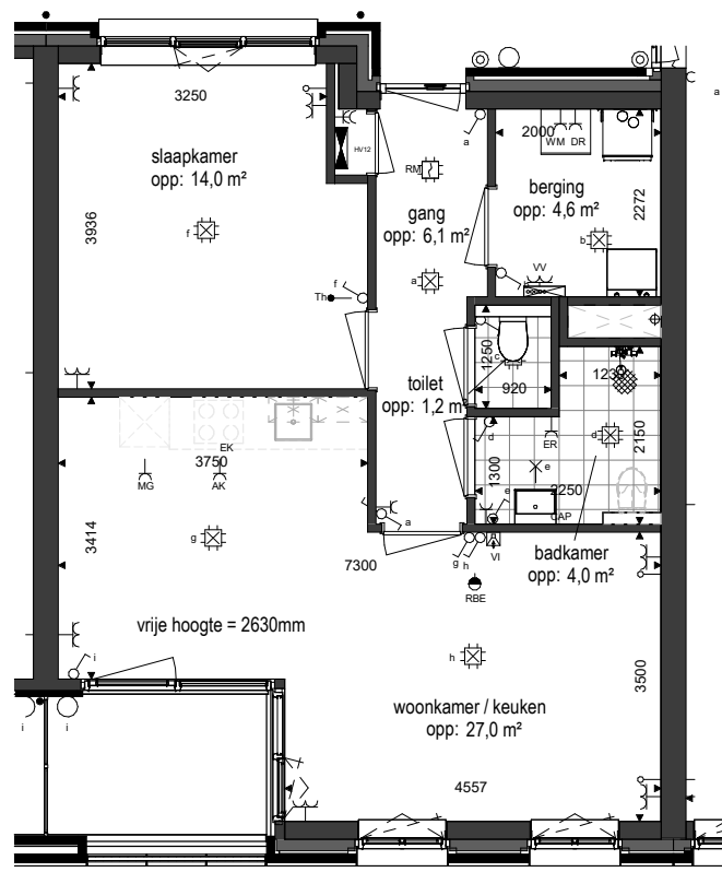
Plattegrond 1 : 100
