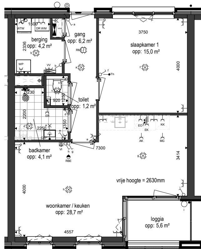
Plattegrond 1 : 100
