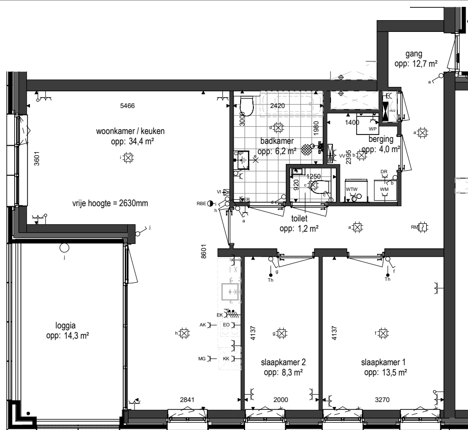
Plattegrond 1 : 100
