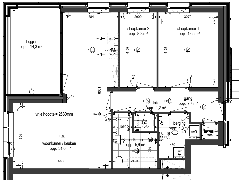
Plattegrond 1 : 100
