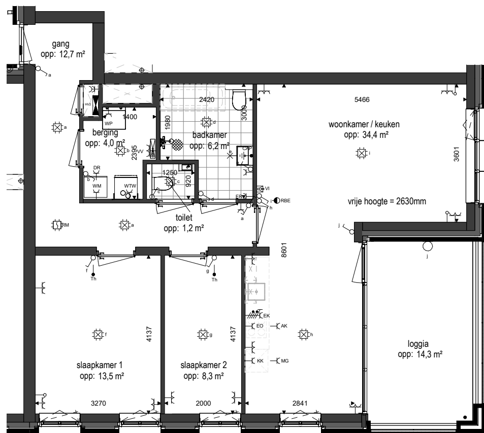
Plattegrond 1 : 100
