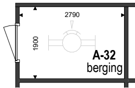
Berging 1 : 100
