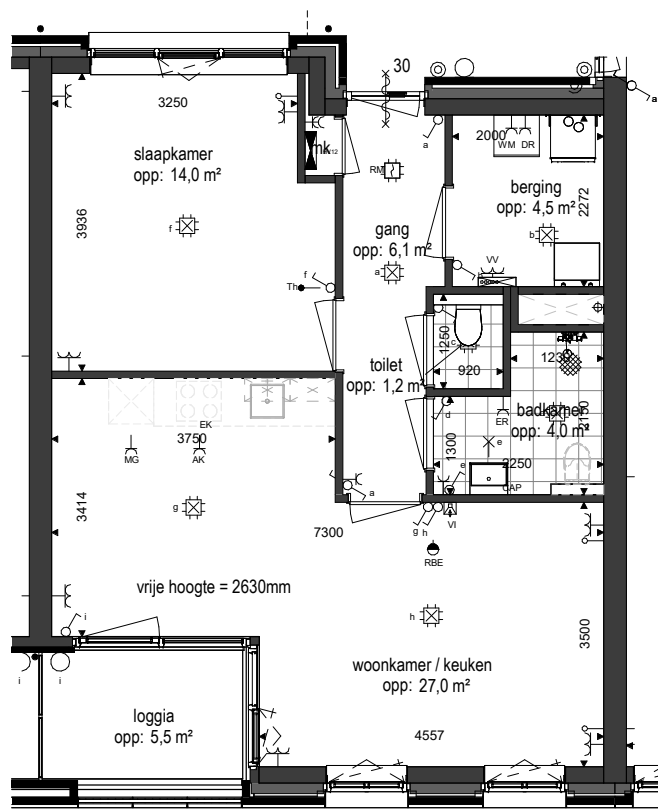
Plattegrond 1 : 100
