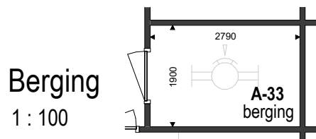
Plattegrond 1 : 100
