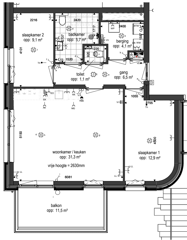
Plattegrond 1 : 100
