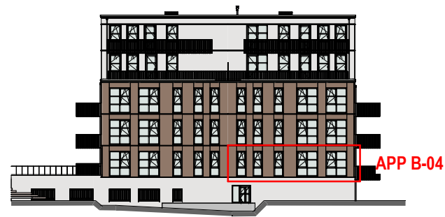
Achtergevel 1 : 500
