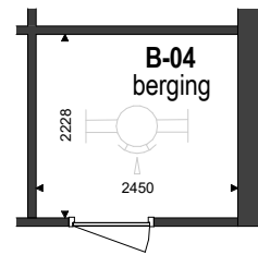
Berging 1 : 100
