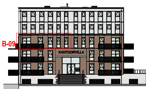
Voorgevel 1 : 500
