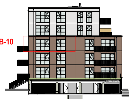
Rechtergevel 1 : 500
