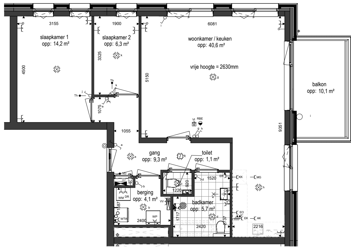
Tweede verdieping 1 : 100
