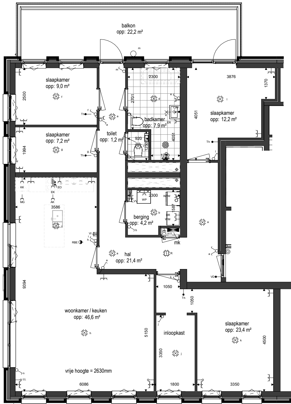
Plattegrond 1 : 100
