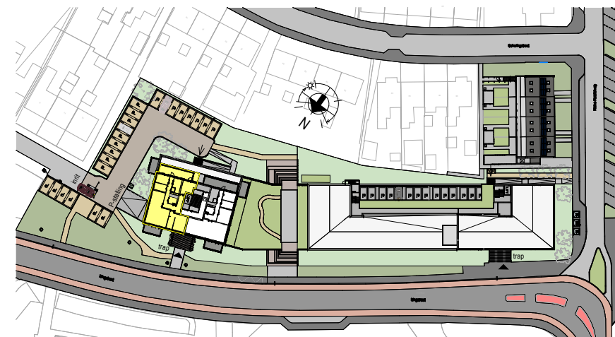
Situatie 1 : 1500
